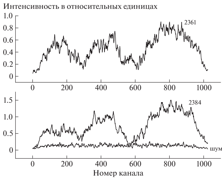
Рис. 2. Спектры индивидуальных импульсов в зависимости от номера канала для базы Аресибо–Грин-Бэнк. Цифрами указаны номера импульсов. Частотное разрешение равно 31.25 кГц, временной сдвиг между спектрами равен 86 с.
