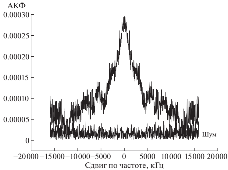
Рис. 6. Частотная ковариационная функция от комплексных кросс-спектров для наземно-космической базы Аресибо-“Радиоастрон”, посчитанная с использованием уравнения (4). Там же приведена соответствующая функция, посчитанная по шумам.
